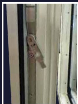
Système anti-fausse manoeuvre et anti-fatigue
