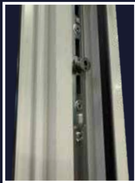
Système sécurité : rouleau champignon anti-dégondage et anti-effraction
