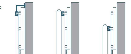
Etrier de guidage fixé sur le pilier
