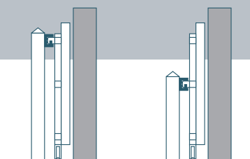
Poteau de refoulement 120/120 mm avec étrier et barre de guidage, fixation basse ou haute.
