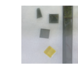
Fusion V8.4
