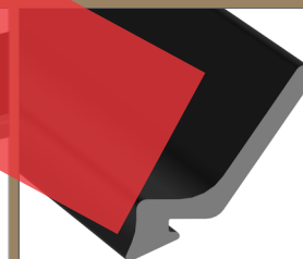
JOINT BIMATIÈRE À EFFET GLISSANT SUR 4 FACES
