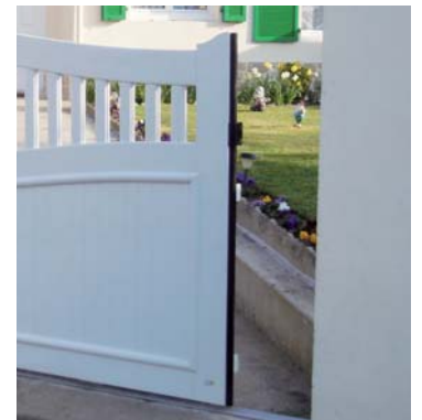
DE SÉRIE Joint en caoutchouc pour absorber l'effort du moteur en cas d'obstacle.
